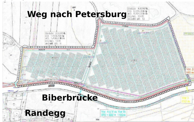
Abb. 2: Vorläufige Modulplanung des Solarparks (16.04.2024, EngCon GmbH).
